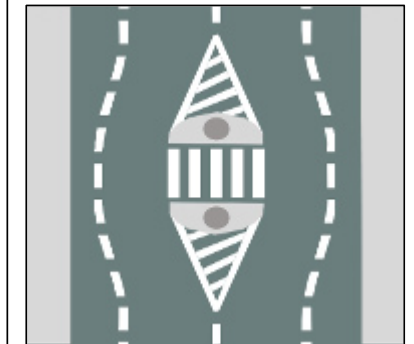
Vorschlag der Anwohner mit Mittelinsel und Angebotsstreifen
