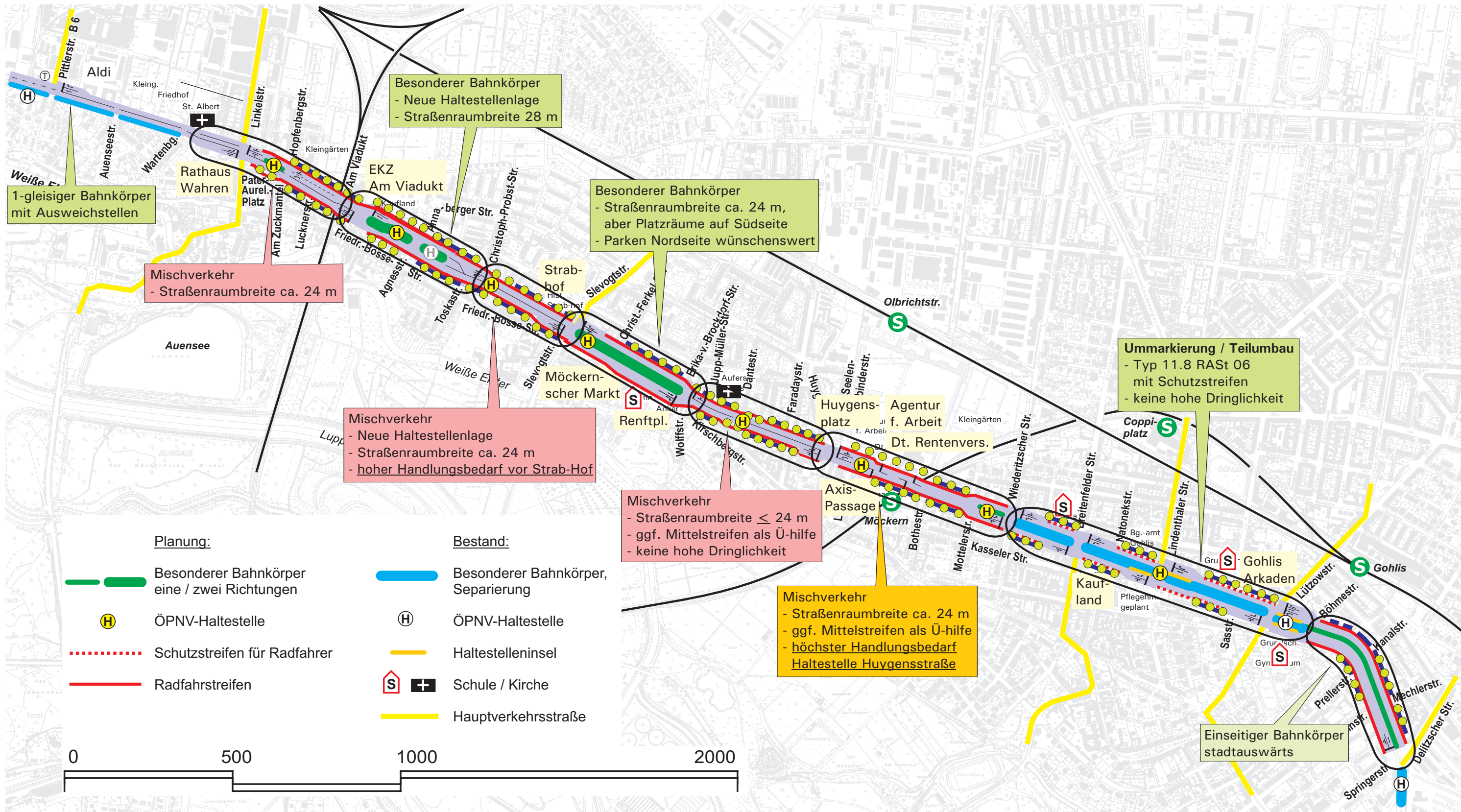
Abb. 67 Zwischen der Stadt Leipzig und den LVB grundsätzlich abgestimmtes Konzept (Stand 07.10.2011)
